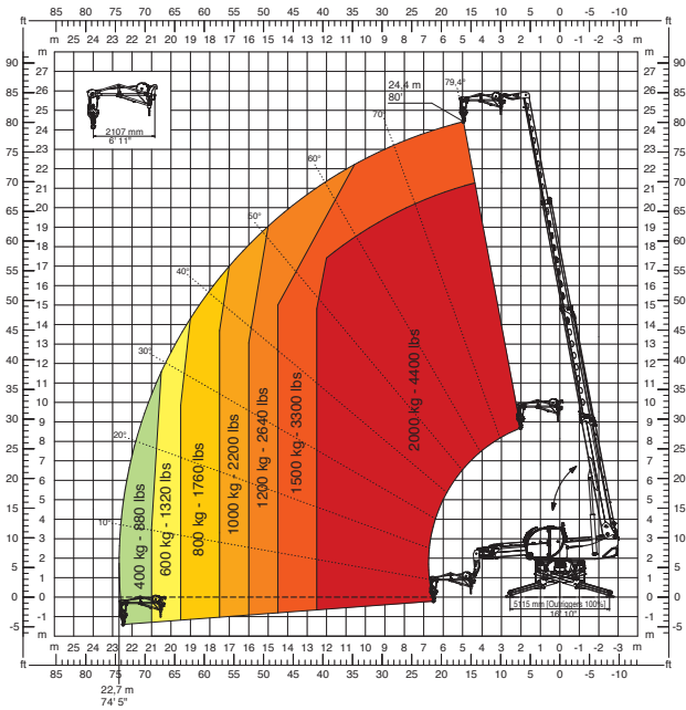
JW 2000 Jib lier 2.000 kg
