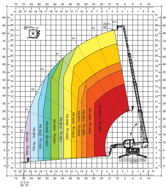
W 3,5 Lier 3,5 t
