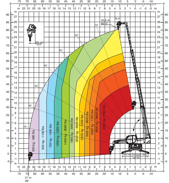
JW 2000 Jib lier 2.000 kg
