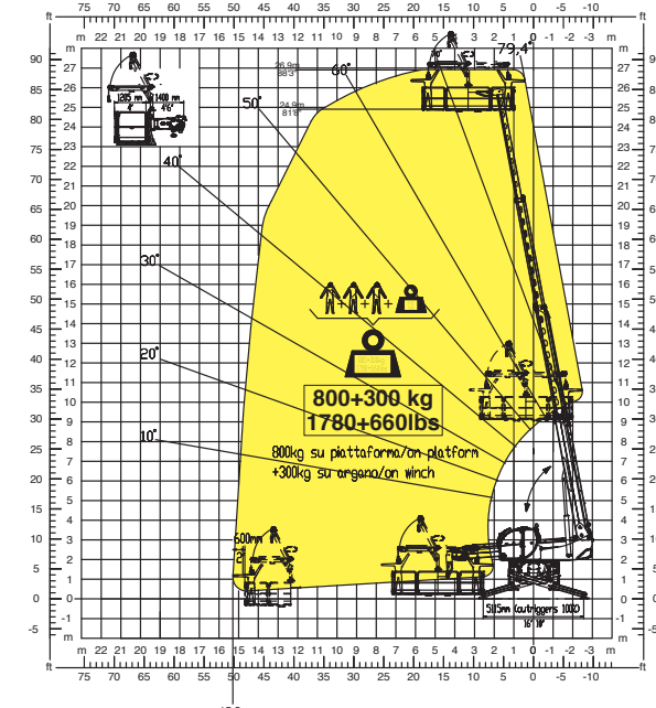
REP 8.2-4,7 W0,3 Werkplatform 4,7 m 800 kg met lier 300 kg
