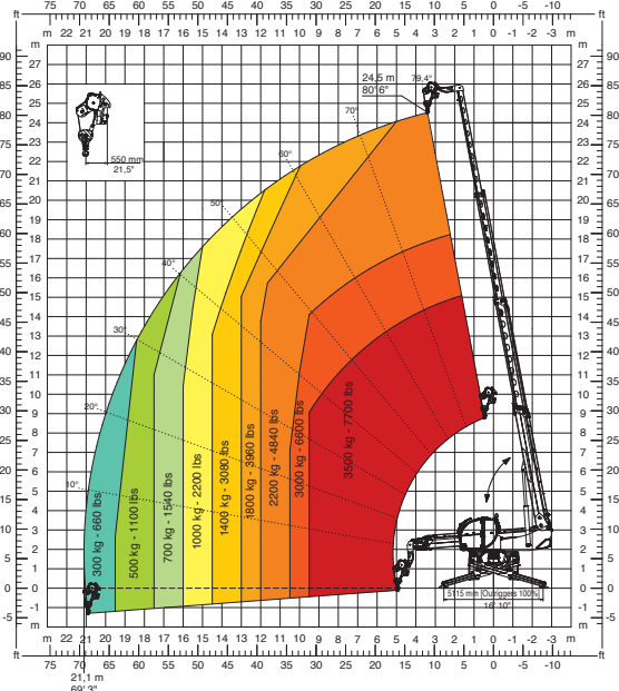
JW 1500 Jib lier 1.500 kg
