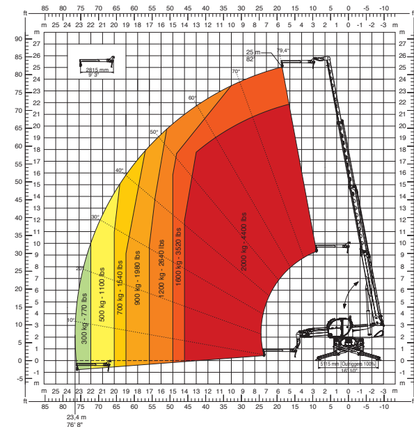
REP 2-4,5 Rotierend uitklapbaar werkplatform 500 kg
