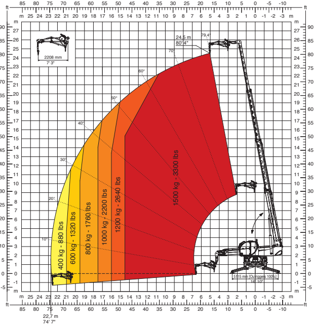
JW 1500 Jib lier 1.500 kg
